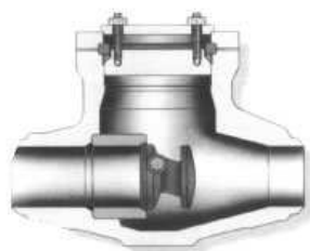
TILTING, CASTELO APARAFUSADO OU SELADO POR PRESSÃO Classes de pressão ASME 600 - 4500, 2 - 24" (50-600 mm)
